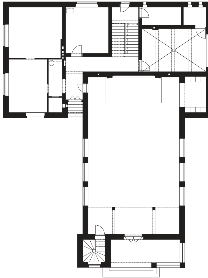
PŮDORYS 1.NP M 1:200 - STAV ⌚
