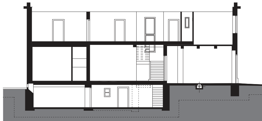
ŘEZ PŘÍČNÝ M 1:200 - STAV
