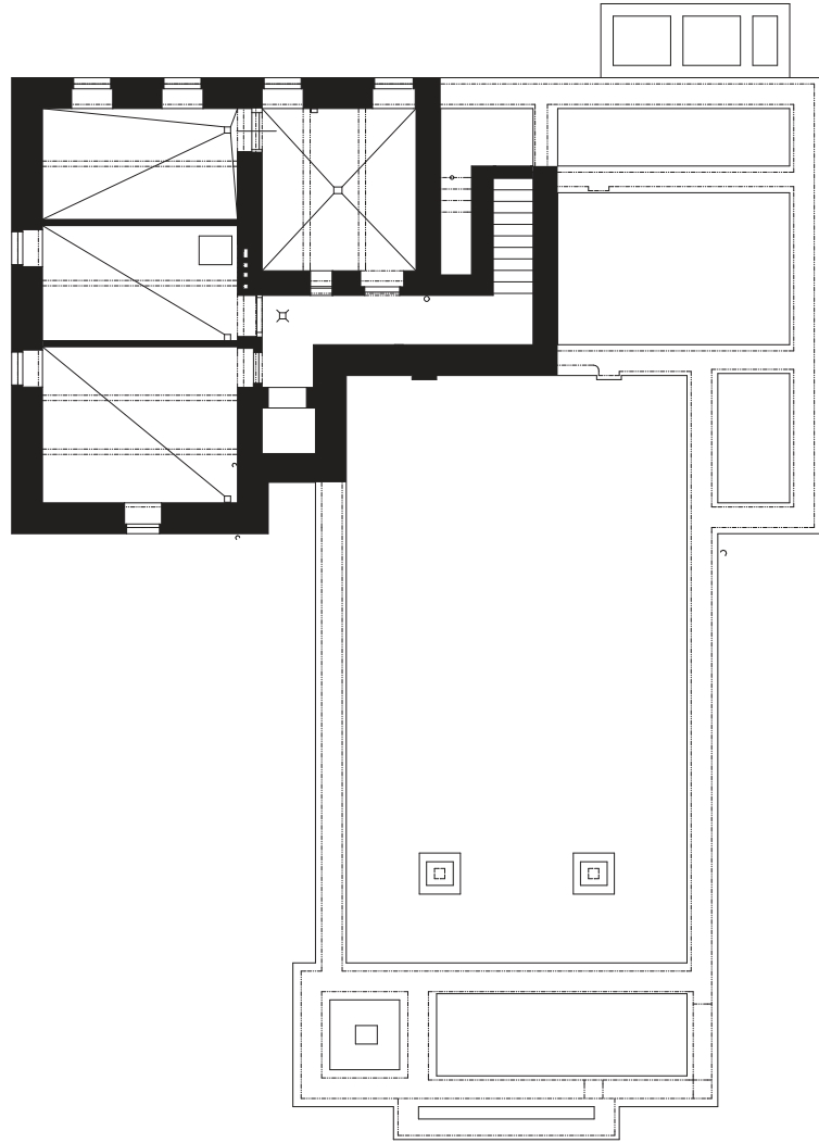
PŮDORYS 1.PP M 1:200 - STAV ⌚
