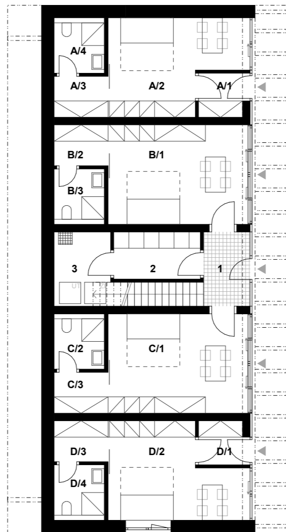
PŮDORYS 1.NP VARIANTA "2"
