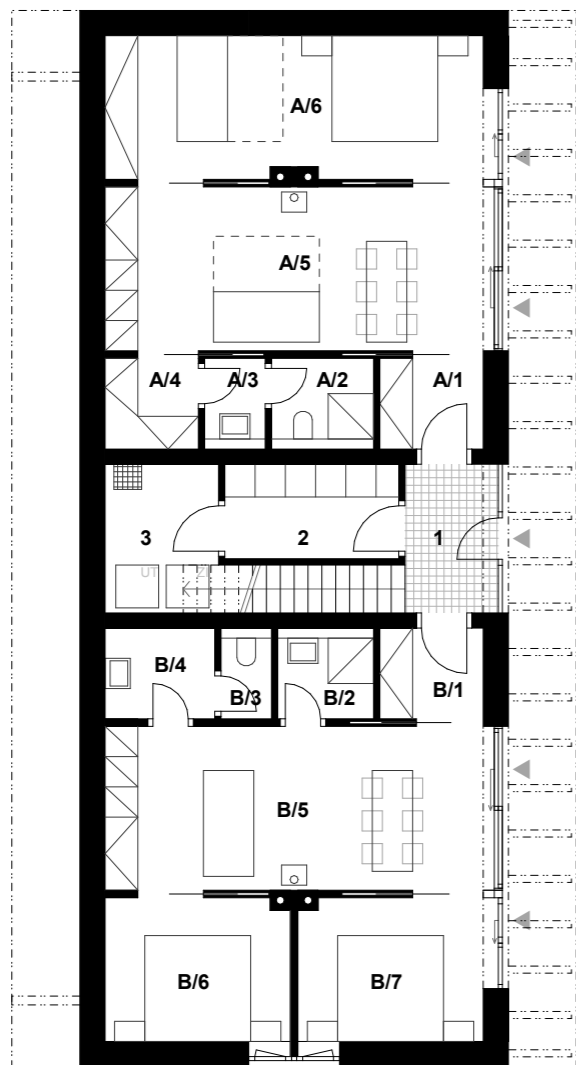
PŮDORYS 1.NP VARIANTA "1"
